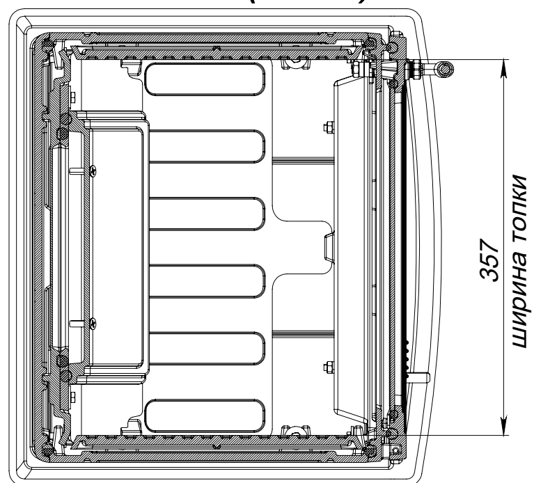
Б-Б (1 : 5)
